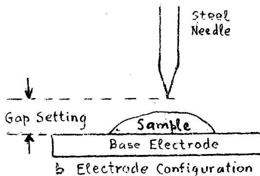
Fig E17 Picatinny Test No 1
